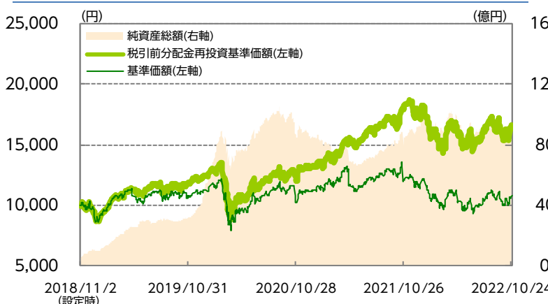
基準価額・純資産の推移 当初設定日（2018/11/2）～2022/10/25 分配の推移（1万口当り、税引前）
